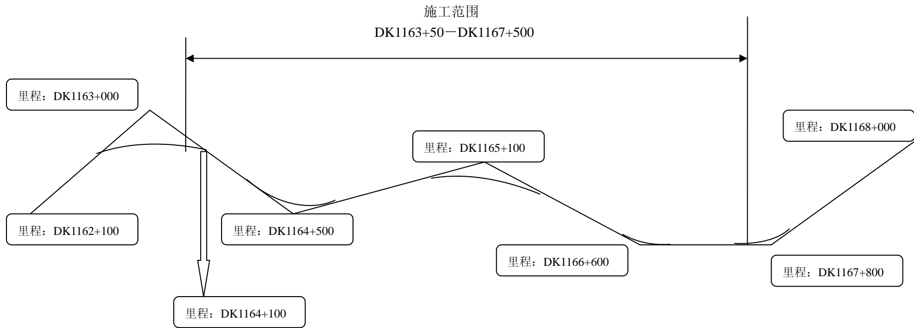
竖曲线示意图
